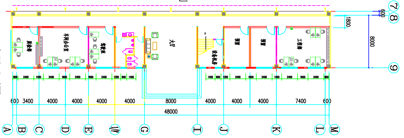
底层平面图 层高4.800
