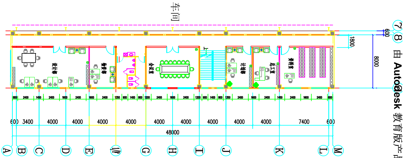
三层平面图 层高4.200
